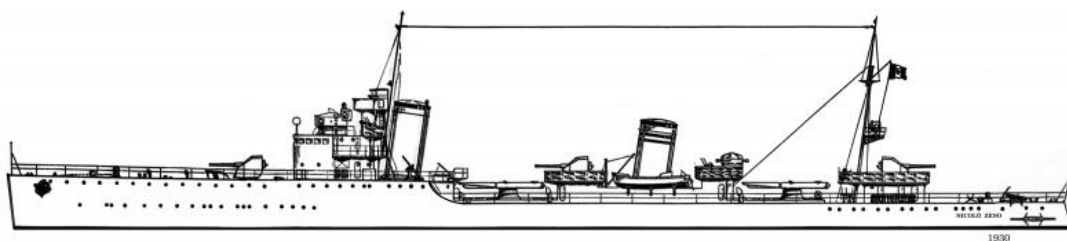
Disposizione degli oblò esploratore NICOLÒ ZENO - Cantieri Navali del Quarnaro Fiume
